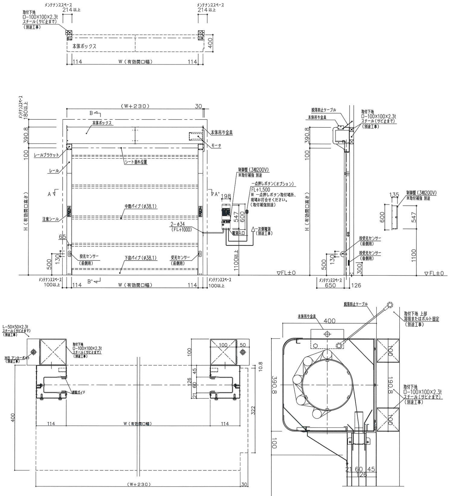
RB-2a, RB-3a 納まり図
